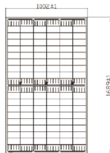
Module Diagram:
